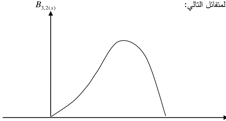
الشكل البياني رقم (3) للتوزيع المعياري B_{3,2}(x)
