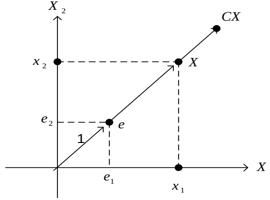
الشكل (1-1) تمثيل وتمديد وتقليص الأشعة في المستوى
